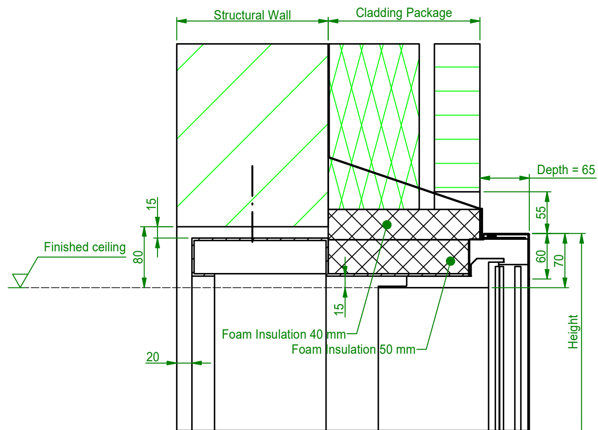
Sheet 3 ( 1 : 5 )
