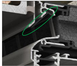
zelfregelende klep elke 10 cm geperforeerd
