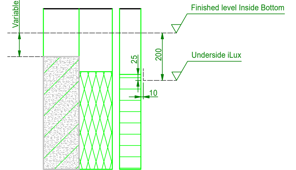
Bottom detail ( 1 : 10 )
