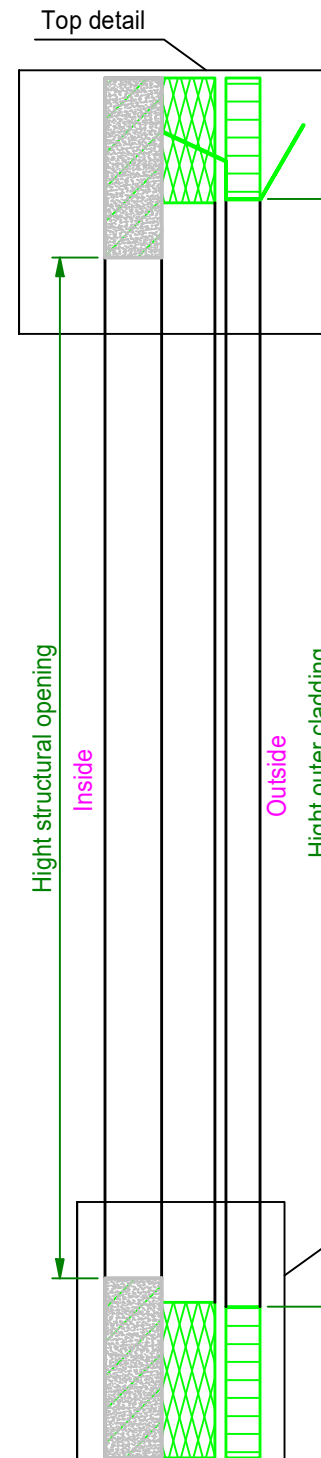
SECTION H-H ( 1 : 20 )
