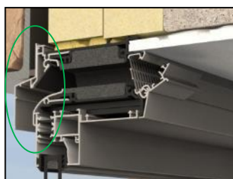
Regenkap Invisivent EVO HR
